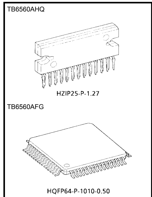
Weight HZIP25-P-1.27: 9.86 g (typ.) HQFP64-P-1010-0.50: 0.26 g (typ.)
